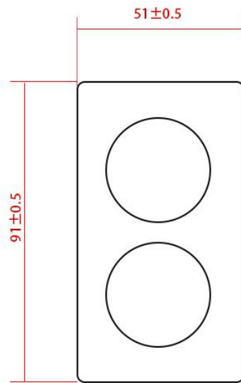
正面 (外壳尺寸)
