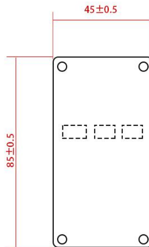
背面 (开槽尺寸)
