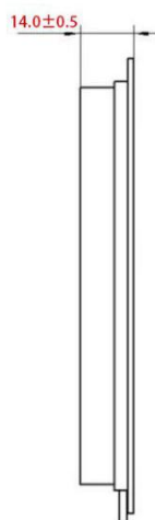
侧面 (配件+支架)
