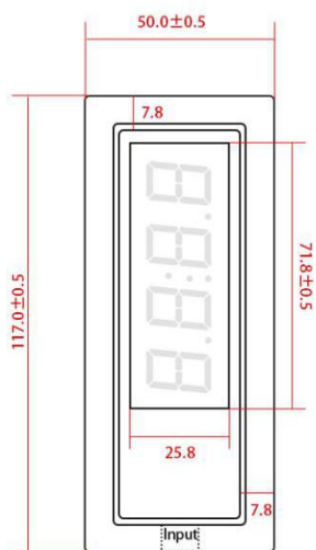
正面 (配件+支架)
