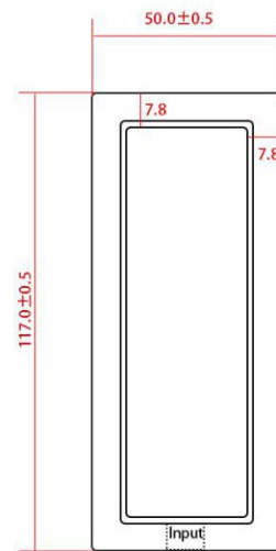
支架
